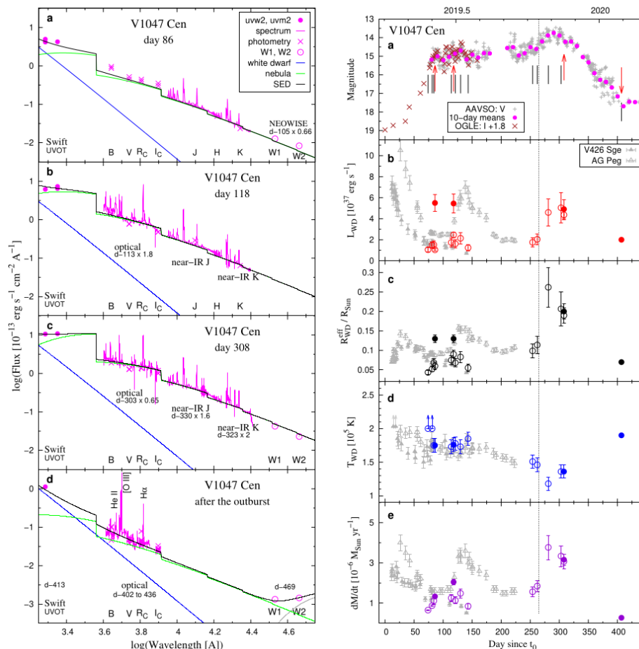
Obr.: Vľavo: Pozorované (magenta) a modelované (čierna čiara) spektrálne rozloženie energie (SED) V1047 Cen vo vybraných dňoch počas jej výbuchu v roku 2019. Vpravo: Vývoj svetelnej krivky V/I (panel (a)) a parametre modelov SED - svietivosť (b), polomer (c), teplota (d) a tempo vyvrhovanej hmoty (e) - počas výbuchu V1047 Cen v roku 2019. Všetky tieto charakteristiky sú typické pre výbuch typu Z And.
